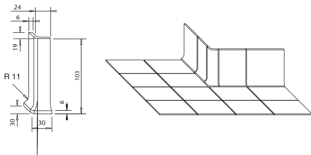
sokl vnější roh | skirting outside corner (GSERCxxx)
