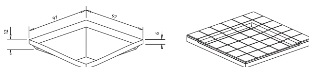
bezbarierová tvarovka rohová | shover piece - corner (GTRONxxx)
