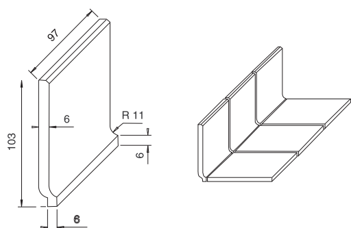
sokl s pozlábkem | cove skirting (GSPOJxxx, GSTONxxx)
