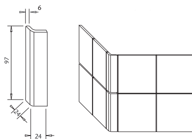
průběžná hrana vnější | shover piece - outside edge (GSEA5xxx)
