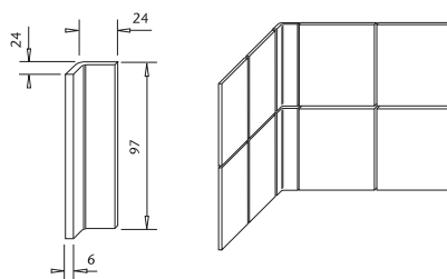
průběžná hrana vnitřní | shover piece - inside edge (GSIA5xxx)
