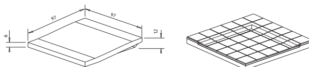
bezbarierová tvarovka průběžná | shover piece - continuous (GTPONxxx)
